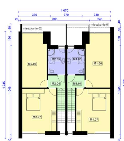
PIĘTRO
